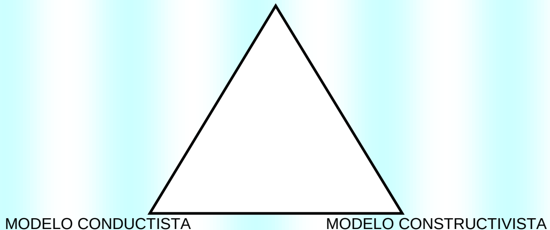
GRÁFICO 1 MODELO COGNOSCITIVISTA
